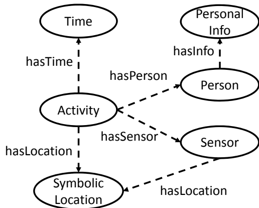
図 2: オントロジの主要概念と関連
