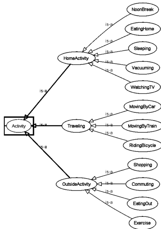
図 3: 行動オントロジ
