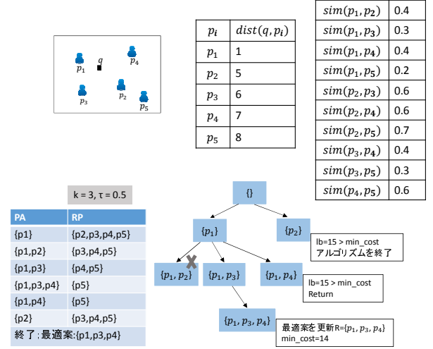
図 2: アルゴリズムの実行例
